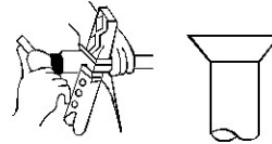
4. Flare pipe.
