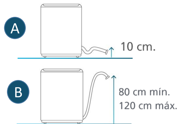
Instalación de manguera de drenado 2
