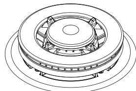
Forma correcta de ensamblar el quemador triple-ring
